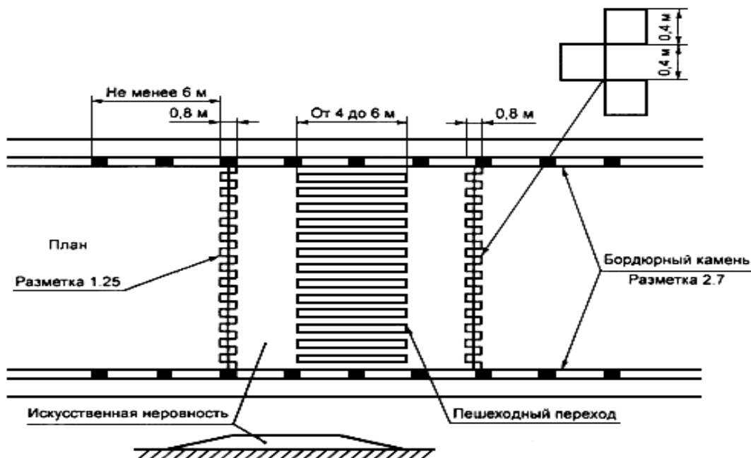
Рисунок 5 - Пример нанесения разметки 1.25 и 2.7 в случае возвышающегося пешеходного перехода, совмещенного с ИН
