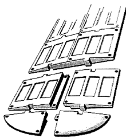
Рис. 3 б - ИН из двух частей основного и краевого элементов
